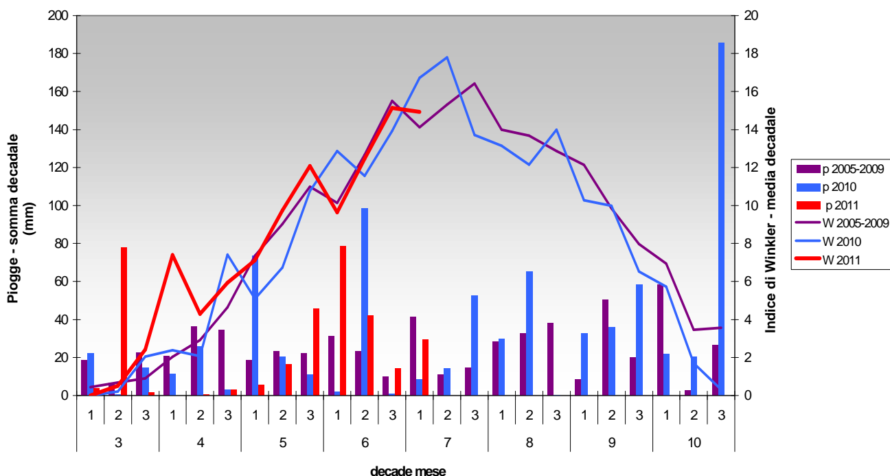
Simione - Precipitazioni e Indice di Winkler media- anni 2005-2010 anno 2010 e 2011
