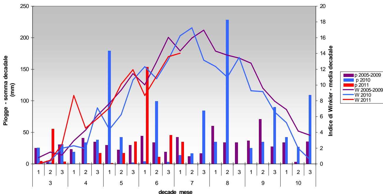
Corte Franca - Precipitazioni e Indice di Winkler - media anni 2005-2010 anno 2010 e 2011
